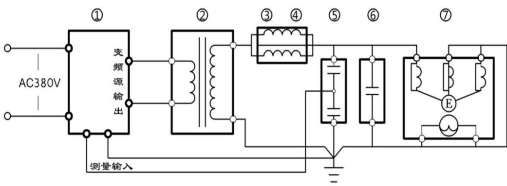
发电机耐压试验接线图
