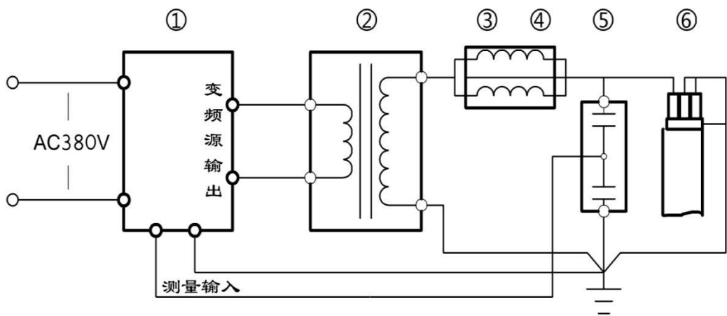
电缆耐压试验接线图
